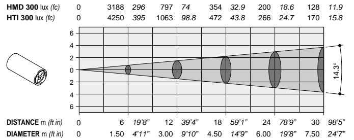
Optional Zoom lens 1:3.5 / 70 mm - Maximum aperture
