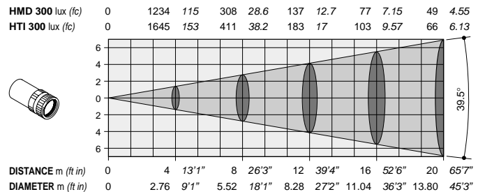
Optional Zoom lens 1:3.5 / 120 mm - Minimum aperture
