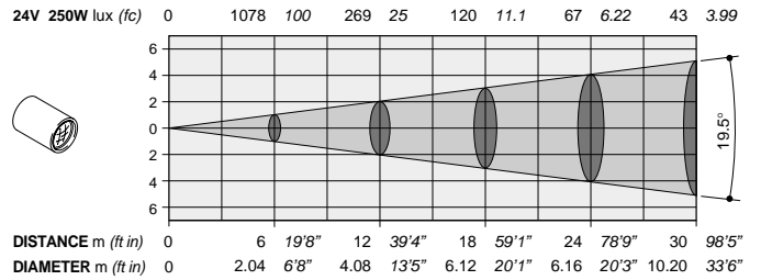
Optional multi-element lens 1:3.5 / 150 mm (19.5°)
