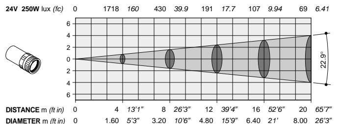
Optional Zoom lens 1:3.5 / 120 mm - Minimum aperture
