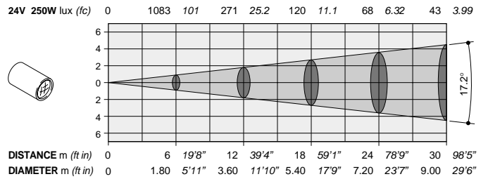
Optional lens 1:4 / 165 mm (17.2°)
