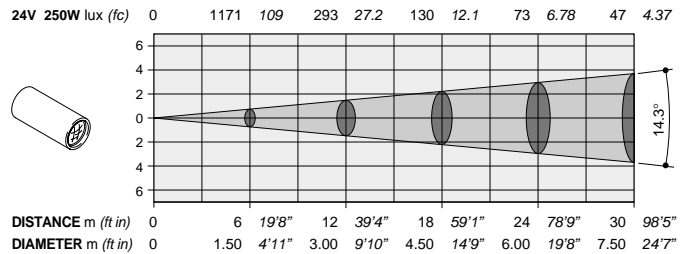
Optional lens 1:4.4 / 200 mm (14.3°)
