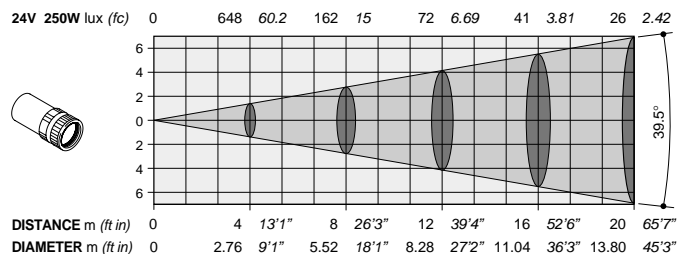
Optional Zoom lens 1:3.5 / 70 mm - Maximum aperture
